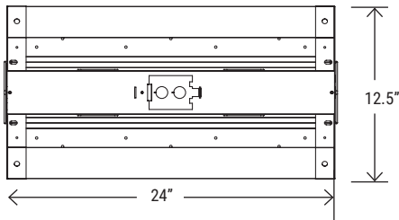
LHB-2FTN-90W / LHB-2FTN-135W
